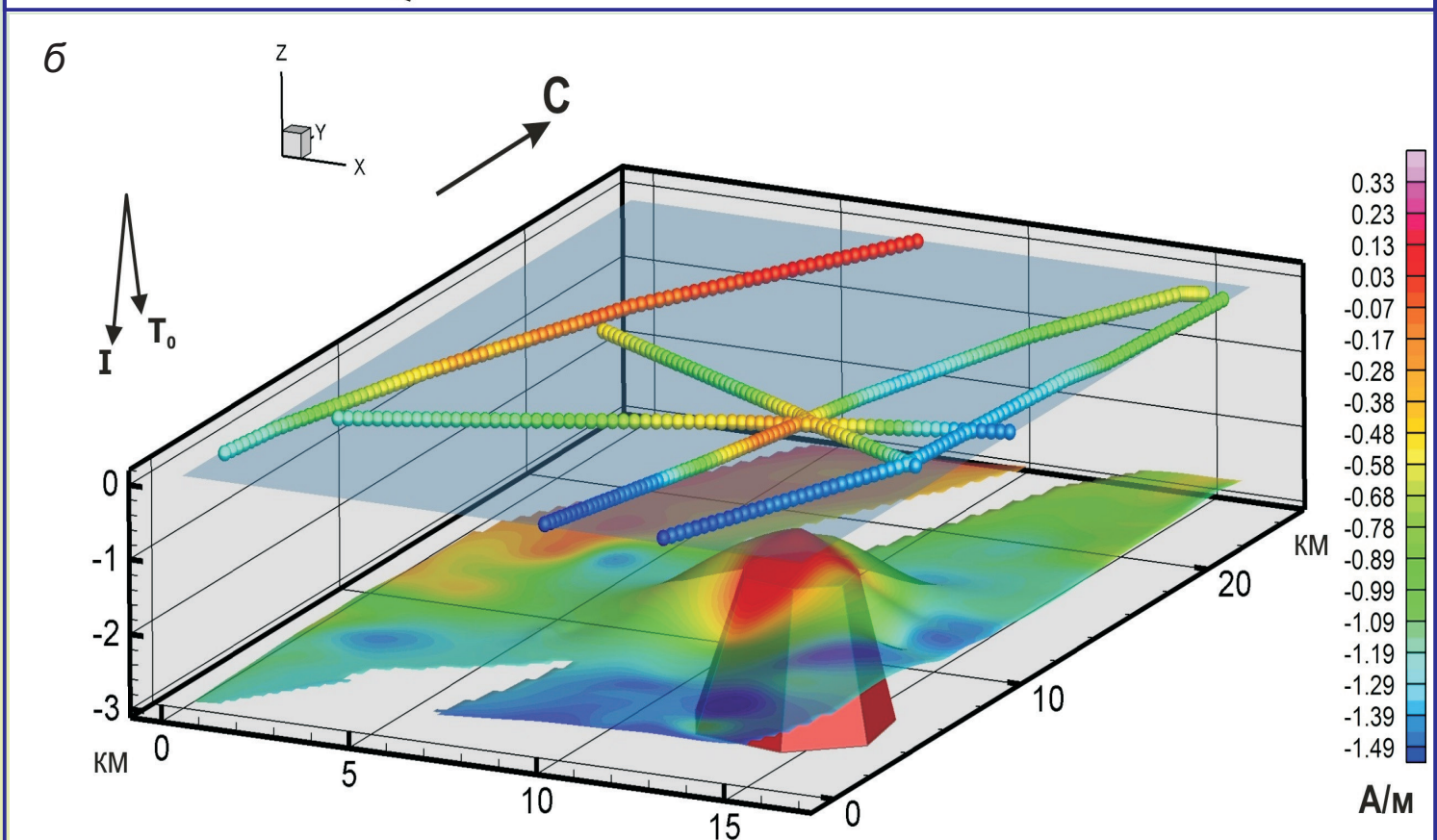
Рис. 2. Примеры интерпретации магнитных аномалий над подводными вулканами КОД с помощью программы ИГЛА: а - вулкан 6.13; б - вулкан Макарова.
