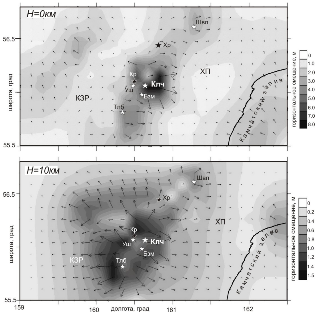
Рис. 6. Распределение горизонтальных смещений на глубинах 0 и 10 км. Стрелками показано распределение модулей векторов смещений. Звездочками показаны вулканы: белыми – действующие, черными – потухшие. Пояснения названий в тексте.
