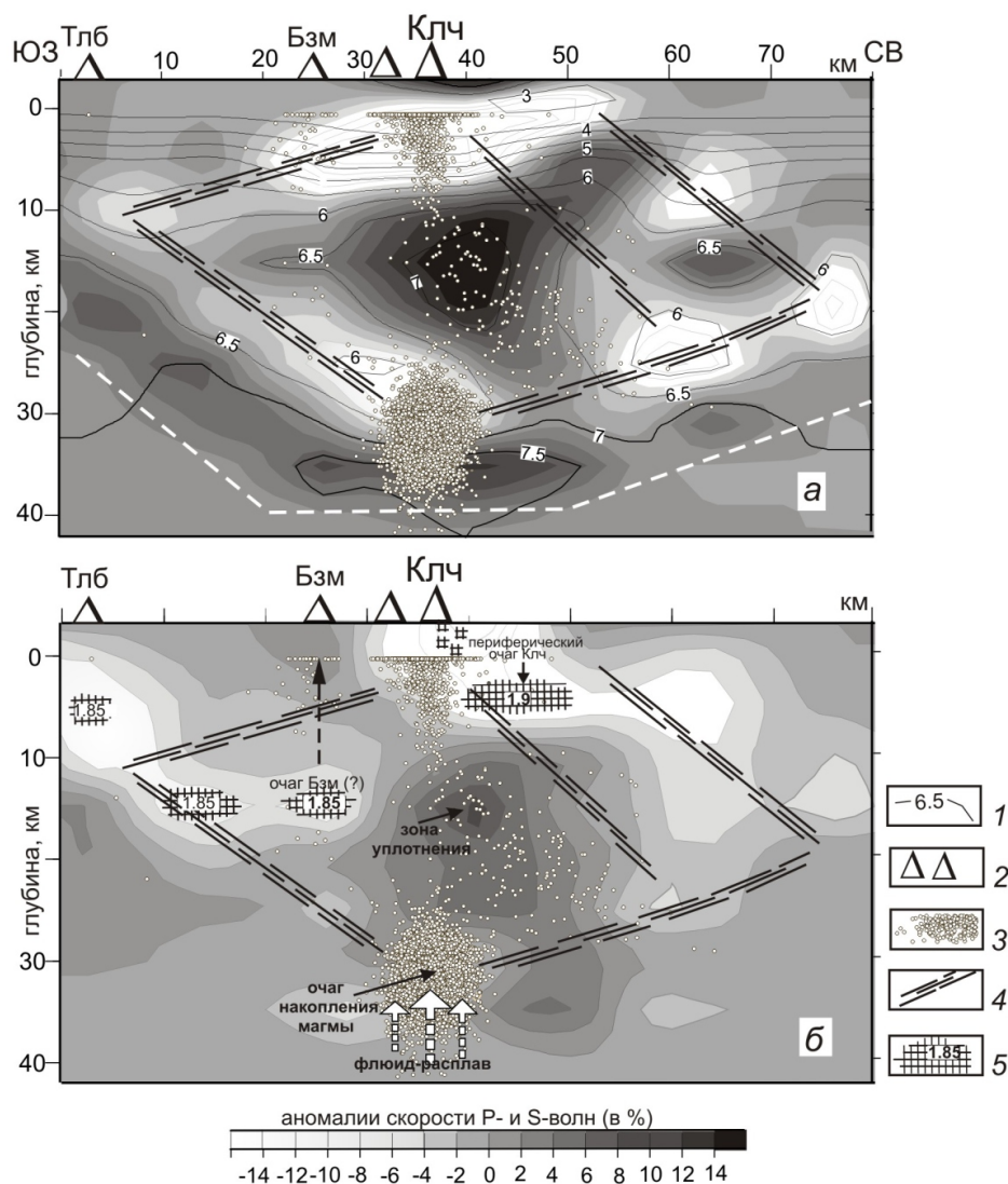
Рис. 8. Тектономагматическая модель встречных ослабленных зон на фоне сейсмотомографического изображения скоростной структуры КГВ в аномалиях V_p (а), V_s (б): 1 – изолинии абсолютных значений скорости V_p (в км); 2 – вулканы; 3 – гипоцентры ВТ землетрясений; 4 – зоны конических и кольцевых ослабленных зон; 5 – магматические очаги; цифры отражают значение параметра V_p/V_s . На разрезе в аномалиях V_p белым штрихом ограничена область высокого разрешения. Остальные пояснения в тексте.
