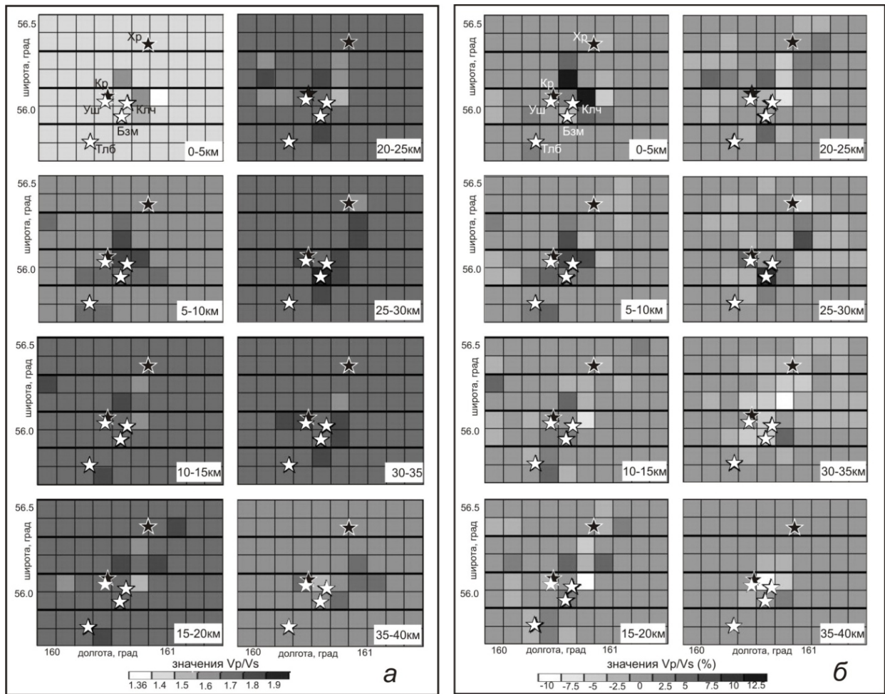
Рис. 5. Схемы распределения значений параметра V_p/V_s для горизонтальных сечений 3D скоростной модели с интервалом 5 км: a – абсолютные значения V_p/V_s ; б – вариации V_p/V_s относительно средних значений в каждом слое. Звездочками показаны вулканы: белыми – действующие, черными – потухшие.
