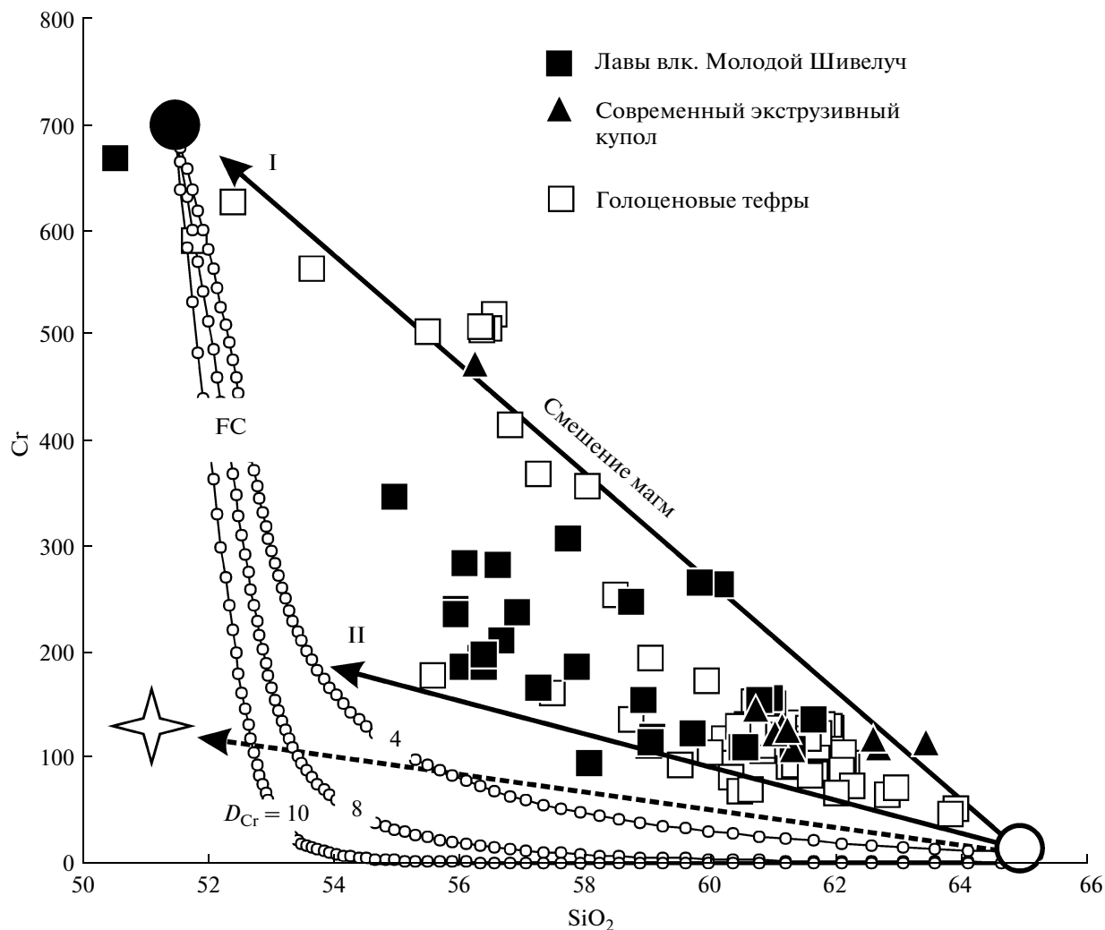
Рис. 17. Вариации содержаний \text{SiO}_2 и Cr в лавах и пирокластических породах вулкана Молодой Шивелуч.
