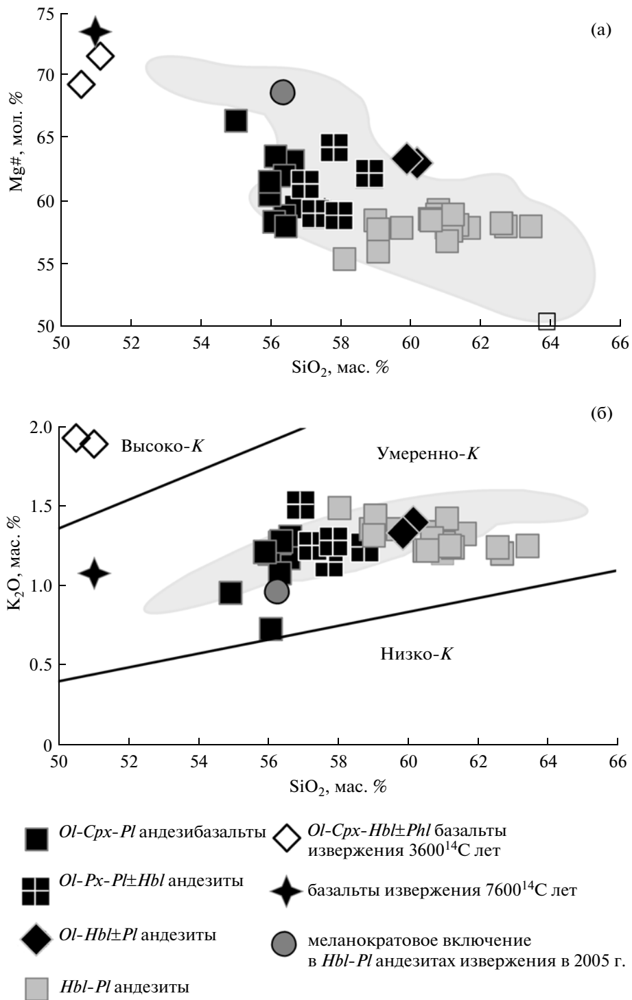
Рис. 13. Состав пород лавового комплекса Молодого Шивелуча в координатах \text{SiO}_2 – \text{Mg\#} (а), \text{SiO}_2 – \text{K}_2\text{O} (б). Состав базальтов извержения 7600 14 С лет, согласно (Вольнец и др., 1997). Серое поле – состав проксимальных пирокластических отложений Молодого Шивелуча (Ponomareva et al., 2007).
