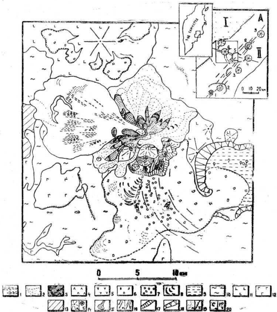
Рис. 1. Схема геологического строения вулкана Тауншиц. 1—5 — лаво-пирокластический комплекс вулкана Тауншиц (поздний плейстоцен-голоцен): 1—отложения направленного взрыва (пунктиром показаны радиальные гряды на их поверхности), 2 — отложения раскаленных лавин (агломератовые туфы), переходящие в аллювиально-пролювиальные отложения подножий, 3 — наслоение лавовых потоков андезитов, андезитобазальтов, составляющих основную постройку вулкана, 4 — лавы андезитов конусов Южный, Монолит, 1 603 м (зона конусов), 5 — лавы андезитов, андезитобазальтов платообразной возвышенности (зоны плато), 6 — морены второй фазы верхнеплейстоценового оледенения, 7—8 — развалы глыб андезитов среди моренных отложений (7 — отдельные горки, 8 — валы), 9 — верхнеплейстоценовые озерные отложения, 10 — верхнеплейстоценовые игнибриты, 11 — среднеплейстоценовые лавы и туфы базальтового, андезитобазальтового, андезитового состава, 12 — нижнеплейстоценовые платобазальты, 13 — плиоценовые туфопесчаники, туфоалевролиты, 14 — центры крупных вулканических построек (а), вулканы на врезке А (б), 15 — лавовые потоки, 16 — сбросы (а), трещины (б), 17 — уступ, ограничивающий платообразную возвышенность (тойю), 18 — эрозийный уступ, ограничивающий Узон-Геизерную депрессию. 19 — восстанавливающиеся границы отдельных порций пирокластического и моренного материала (а), конечноморенные гряды (б), 20 — кратеры и кальдеры на врезке А (а), термальные поля кальдеры Узон (б).
