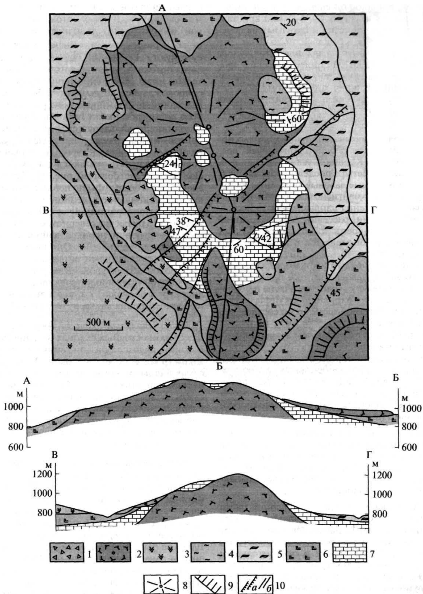
Рис. 7. Схема геологического строения купола Кулакова.
