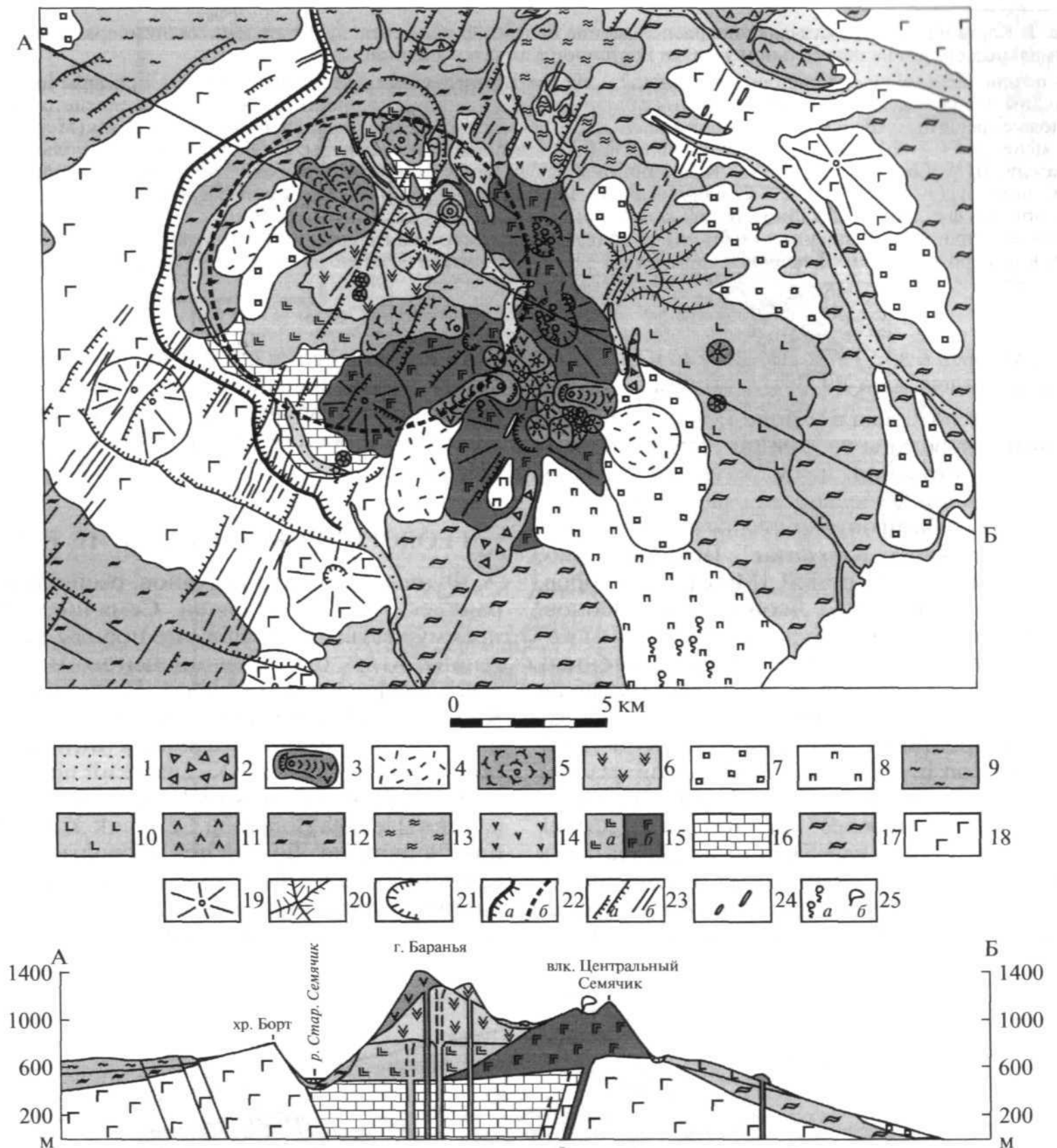
Рис. 3. Схематическая геологическая карта вулканического массива Большой Семячик.
