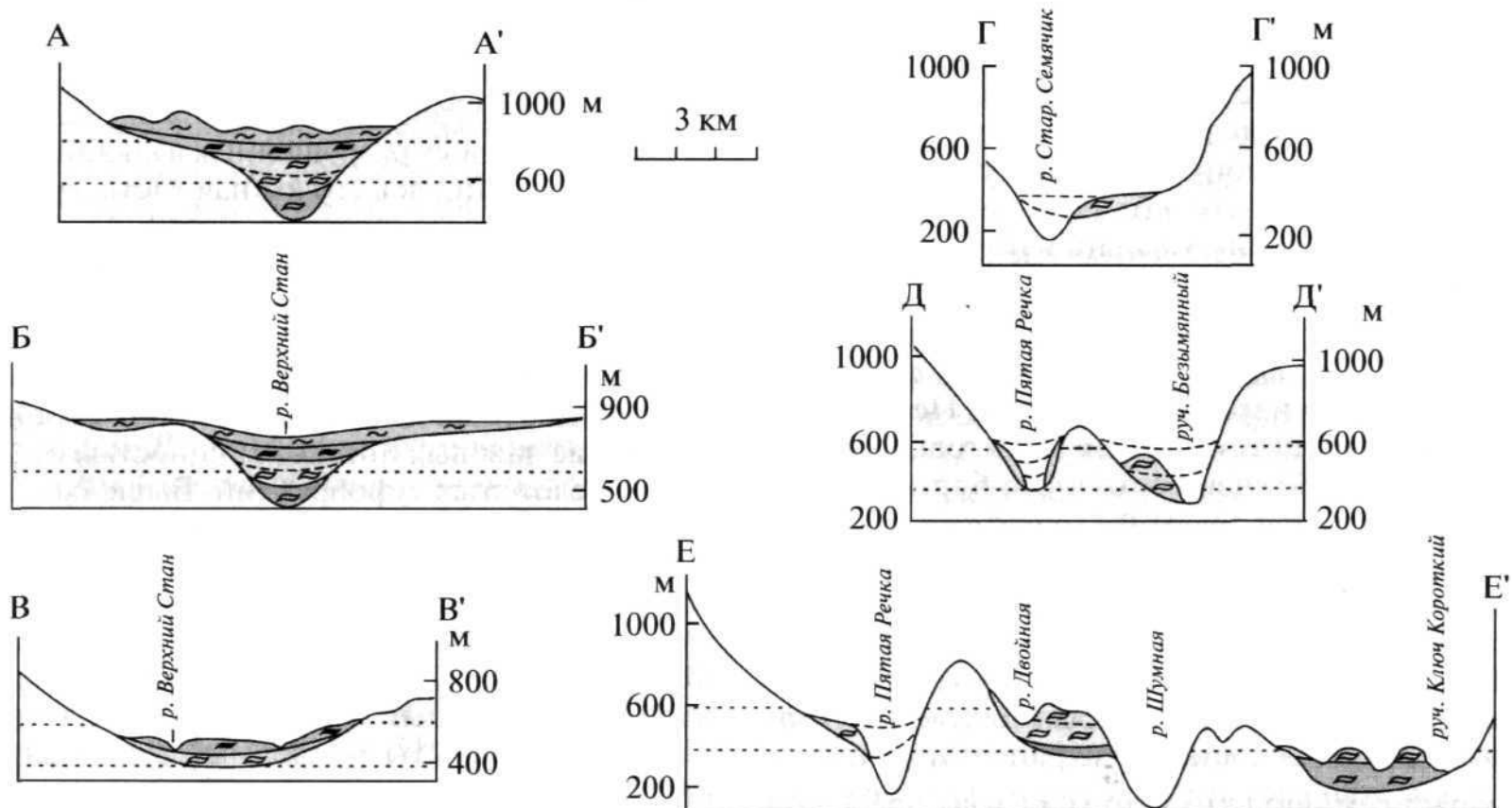
Рис. 5. Схема распространения пирокластических потоков, связанных с образованием кальдеры вулканического массива Большой Семячик (вверху) и разрезы, построенные вкрест простирания отдельных потоков (внизу).
