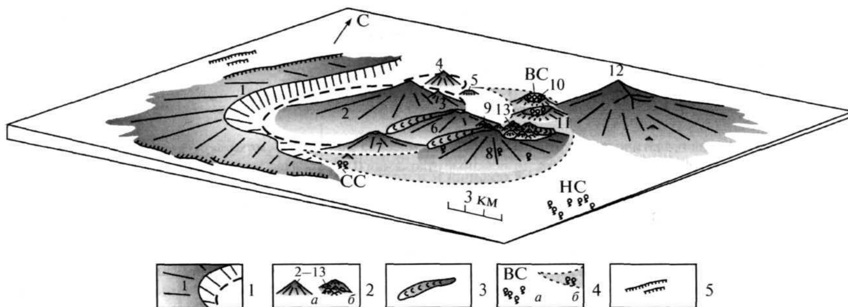
Рис. 2. Блокдиаграмма вулканического массива Большой Семячик.
